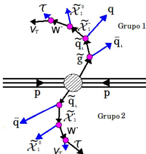
Figura 3.1: Grupos canal de decaimiento, fuente de esta investigación.
