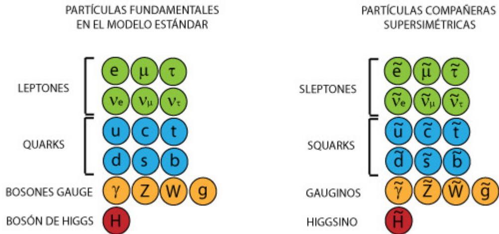
Figura 1.2: Partículas ME y SUSY, Fuente: URL: http://www.ramanujan25449.blogspot.com/2013/01/susy_6764.html
