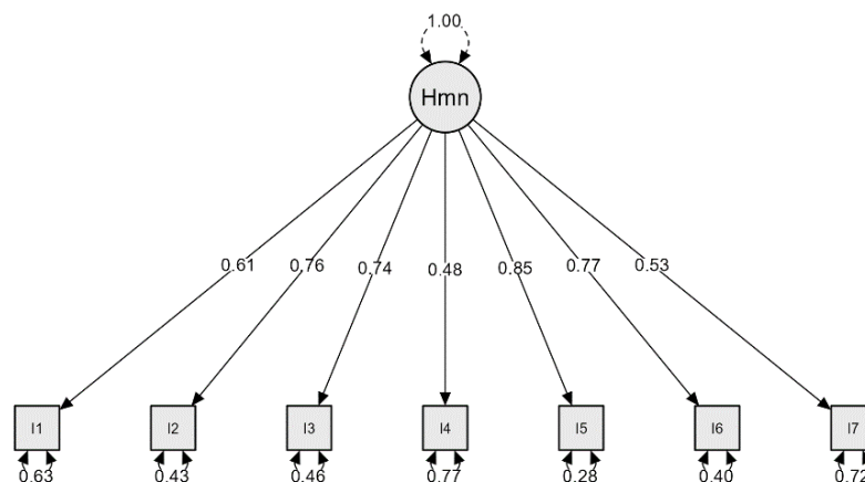
Diagrama de trayectoria - CFA
