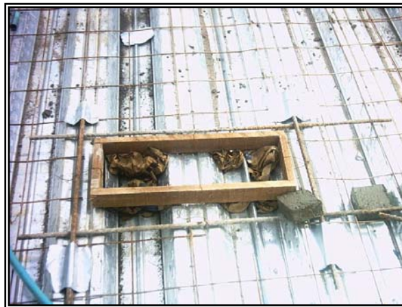
Figura 100. Refuerzo corte buitrones.
