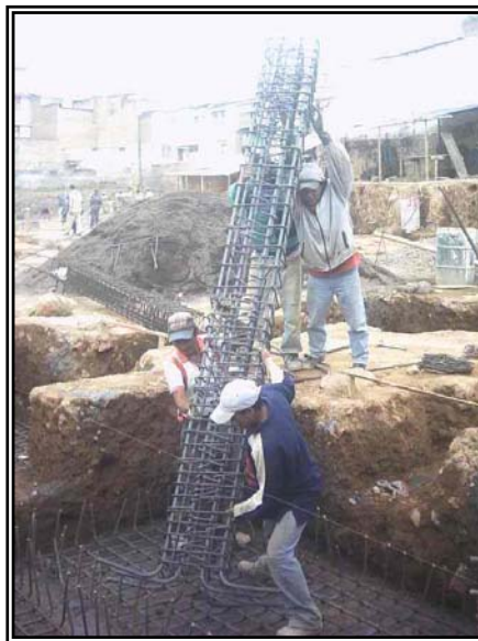
Figura 40. Colocación castillo columnas.
