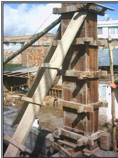
Figura 91. Encofrado y apuntalamiento columnas nivel N+0,00 bloque 6.
