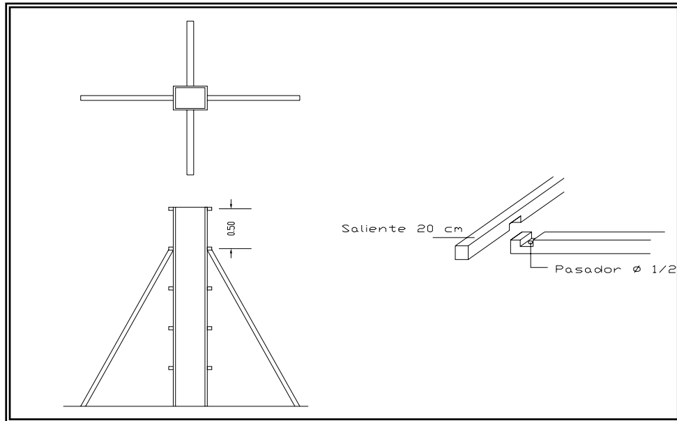
Figura 51. Encofrado y apuntalamiento de columnas
