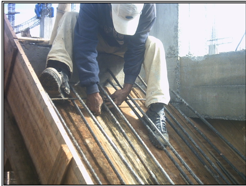
Figura 82. Dovelas para escalera.
