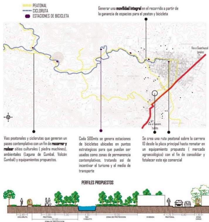
Figura 31. Perfil vial propuesto
