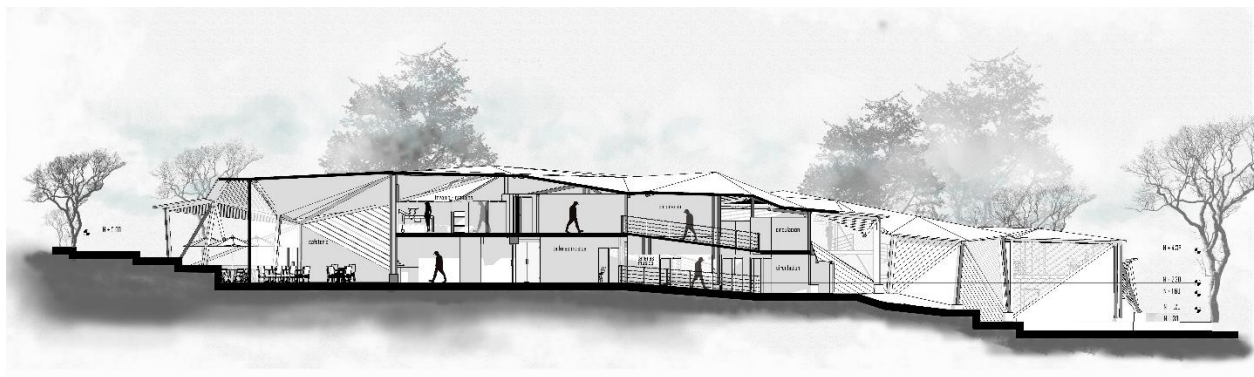
Figura 46. Corte B – B. Fuente : Elaboración Propia
