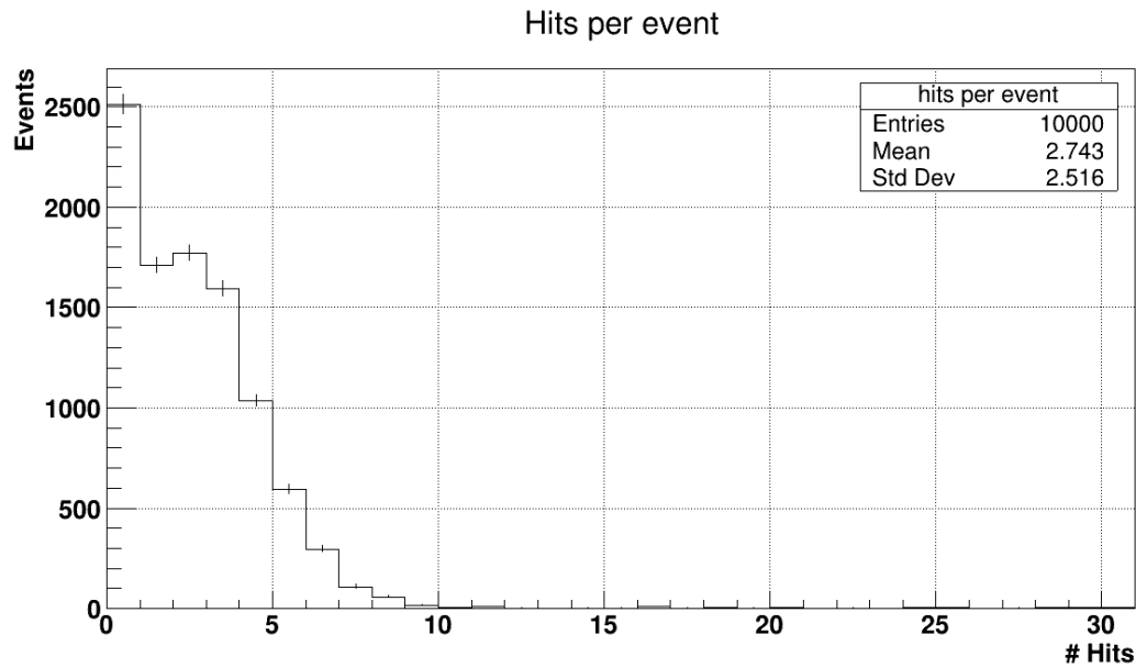
Figura 7.18: Número de impactos por evento generados por los fotones ópticos arriando al fotocátodo del SiPM con QE = 20\%
