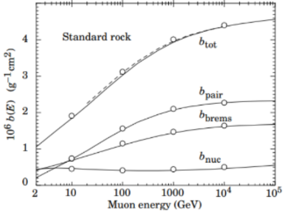
Figura 4.3: Valores de ajuste del termino b(E) asociado a procesos radiativos para muones en roca estándar (densidad \rho = 2,6 \text{ g/cm}^3 ). b_{tot} = b_{par} + b_{brems} + b_{nuc} . [13]
