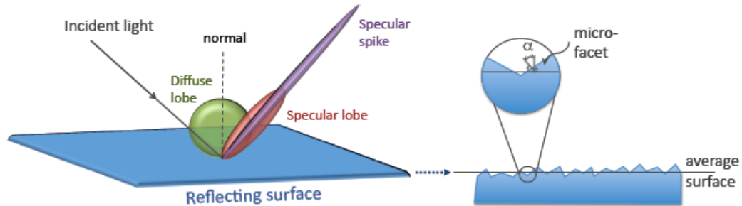
Figura 6.4: Tipos de reflexión y microfacetes[34]
