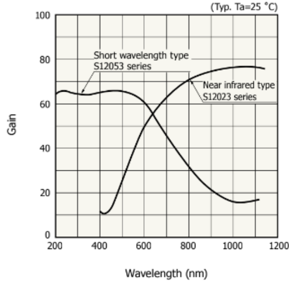
Figura 4.17: Dependencia obtenida de la longitud de onda de la luz incidente para dos APD de Hamamatsu[26]
