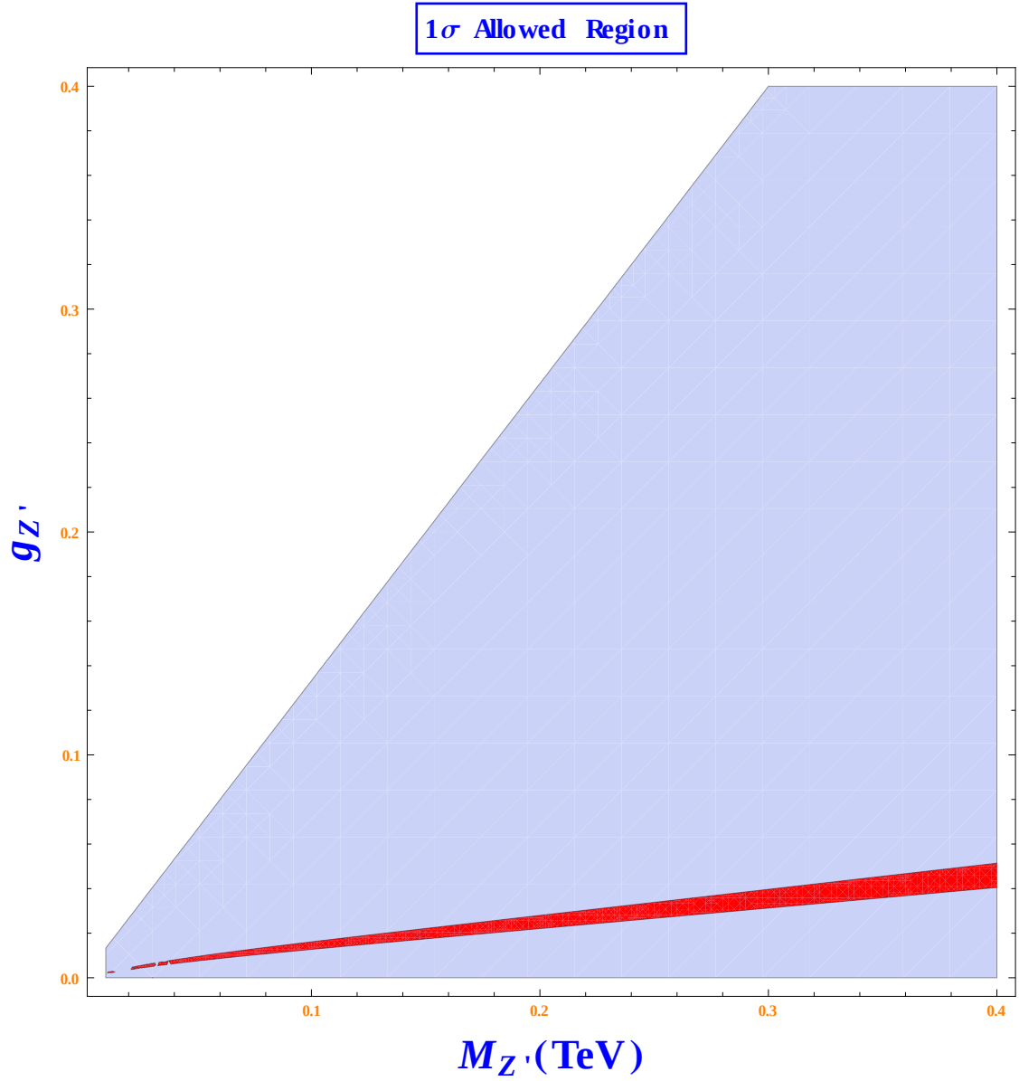
Figura 4.2: La región en rojo corresponde al espacio de parámetros permitido para g - 2 con un nivel de confianza de 1\sigma . La región púrpura es la región permitida por producción tridente del neutrino m_{Z'}/g_{Z'} > 0,75 TeV. Se asume para la masa de la partícula exótica un valor de 80 GeV.
