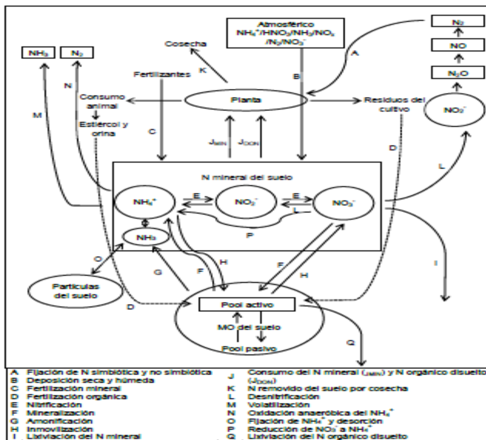
Figura 9. Representación esquemática del ciclo del N en el suelo. Fuente: Stark y Richards (2008).
