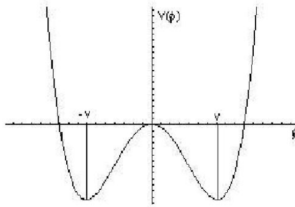
Figura 2: Potencial efectivo para \mu^2 < 0 .
