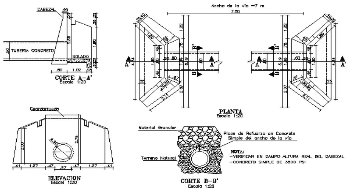
Figura 3.13. Diseño alcantarilla tipo.
