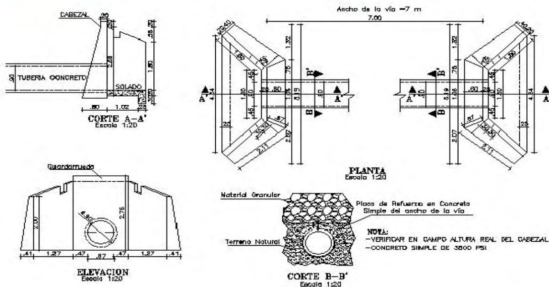
Figura No. 3. Diseño de Alcantarilla Tipo
