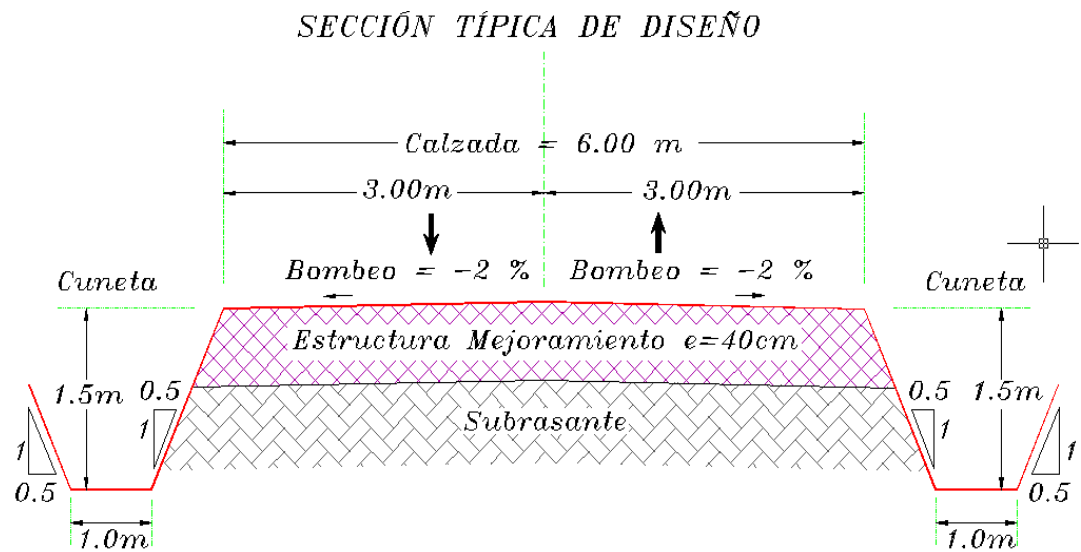
Figura 2.5. Sección típica de diseño.
