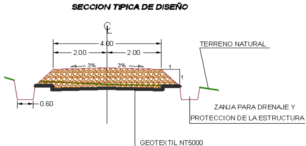
Figura 3.4. Sección típica de diseño.
