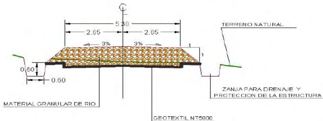
Figura No. 2. Sección Transversal Típica de la Vía.
