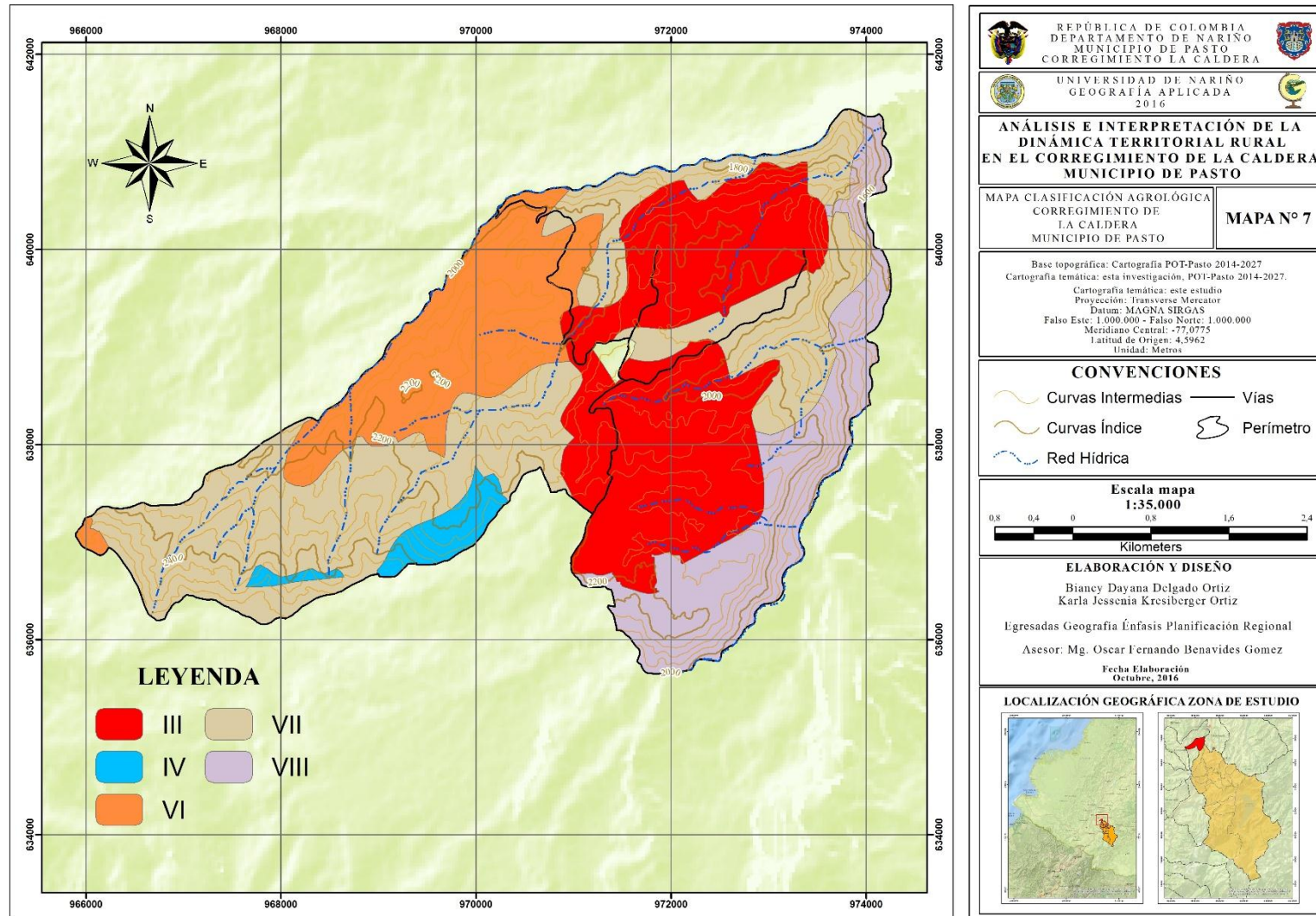
Mapa 7. Clasificación Agrológica
