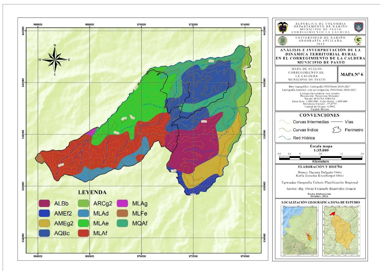
Mapa 6. Suelos
