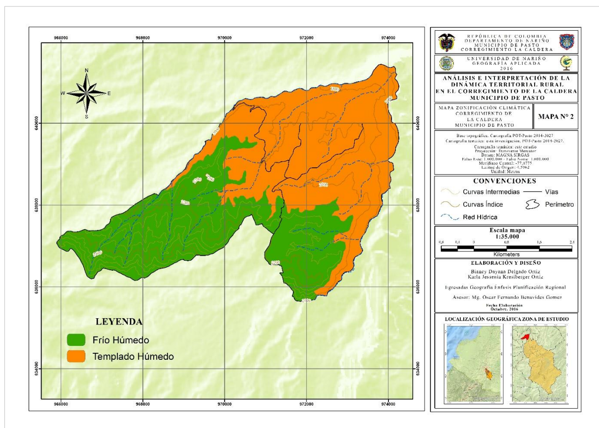
Mapa 2. Zonificación Climática
