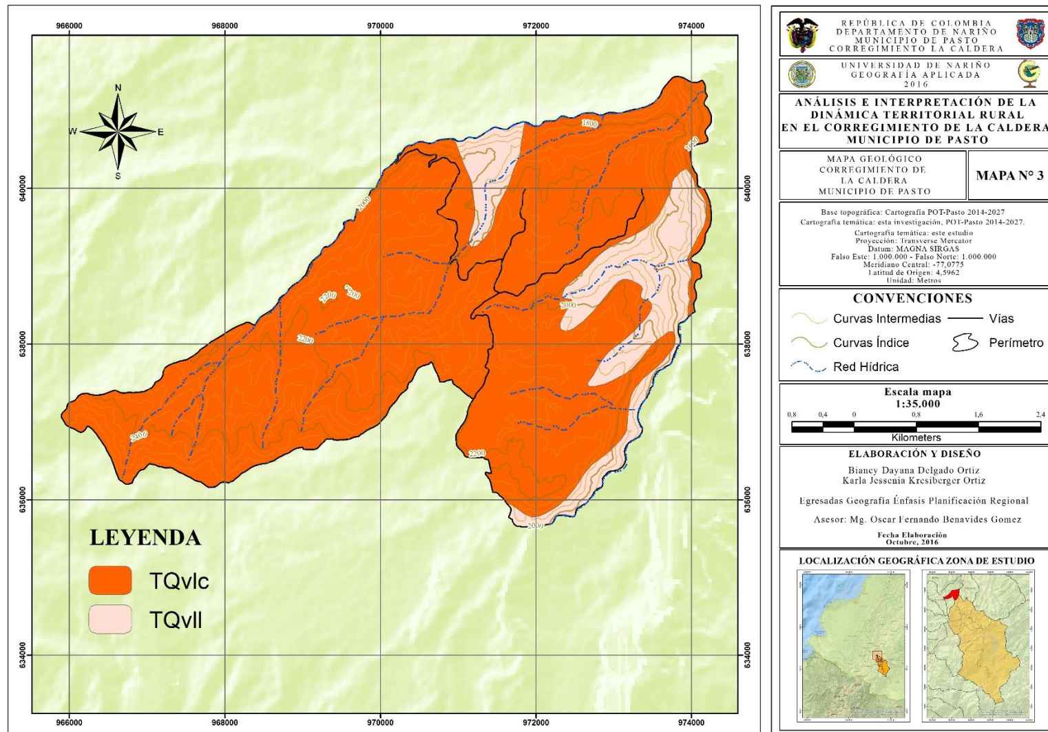
Mapa 3. Geológico
