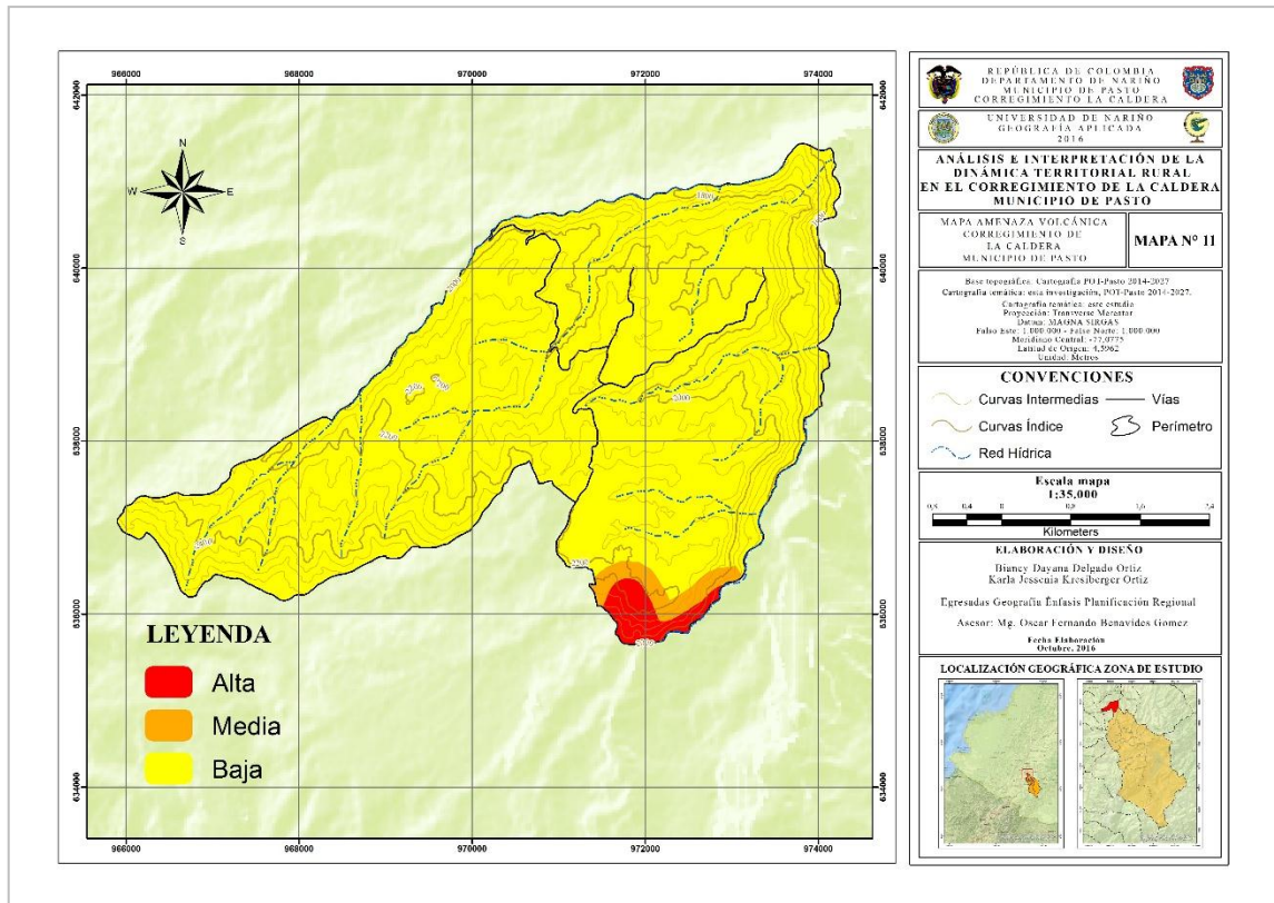
Mapa 11. Amenaza volcánica
