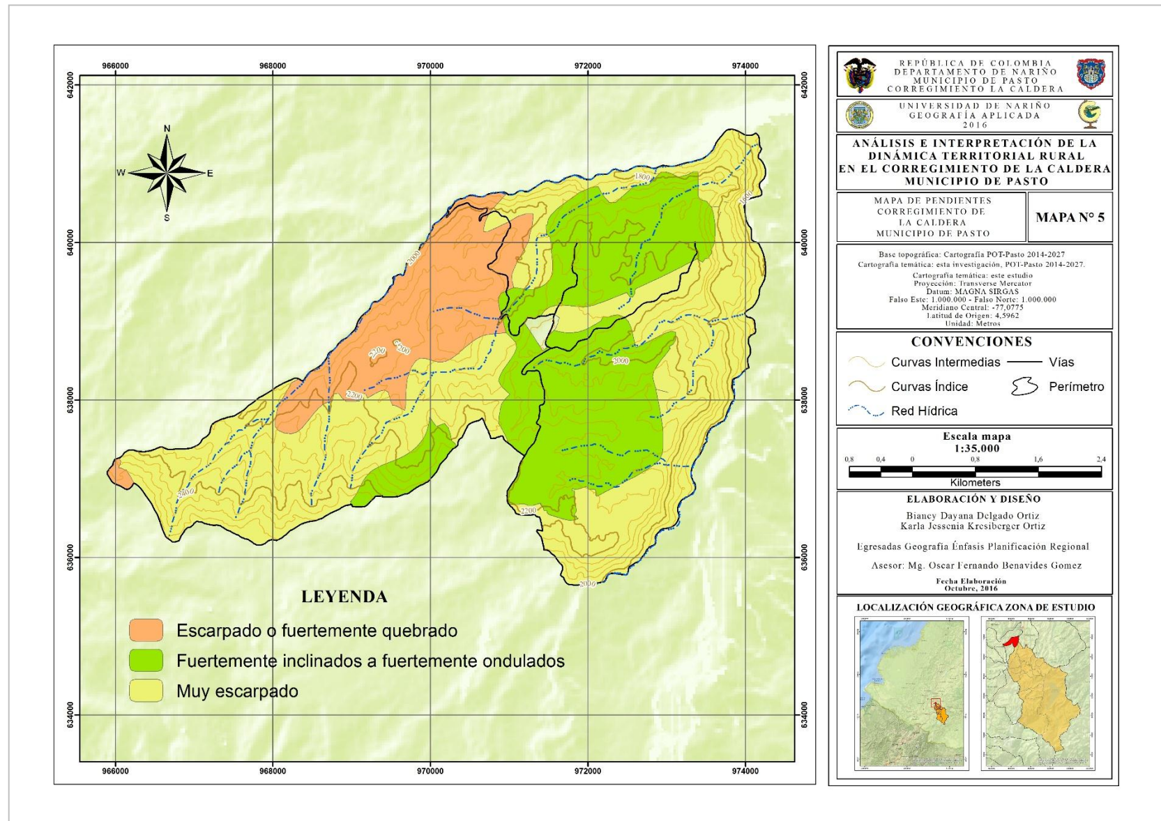
Mapa 5. Pendientes
