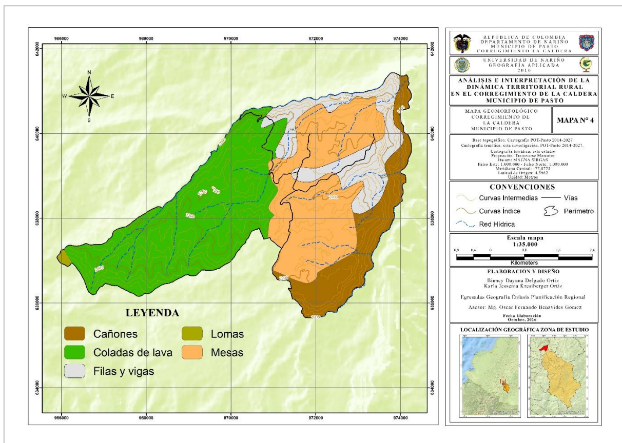
Mapa 4. Geomorfológico
